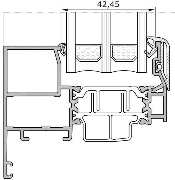
GİZLİ KANAT İÇİN CAM ÇITASI VE FİTİL TABLOSU / GLAZING BEAD AND GASKETS TABLE FOR HIDDEN VENT
