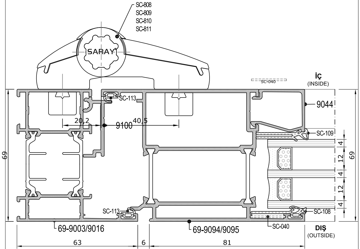
İÇE AÇILIR HEMİYÜZ KAPI
