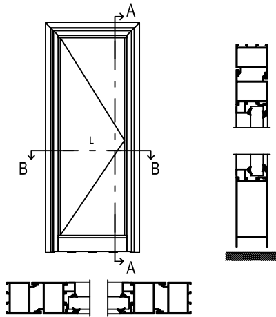
B-B KESİTİ
